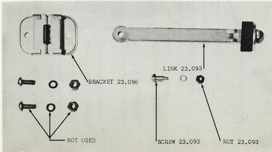
GROUP 23 - FIG. 13 - REAR DOOR CHECK LINK 10-20-80
